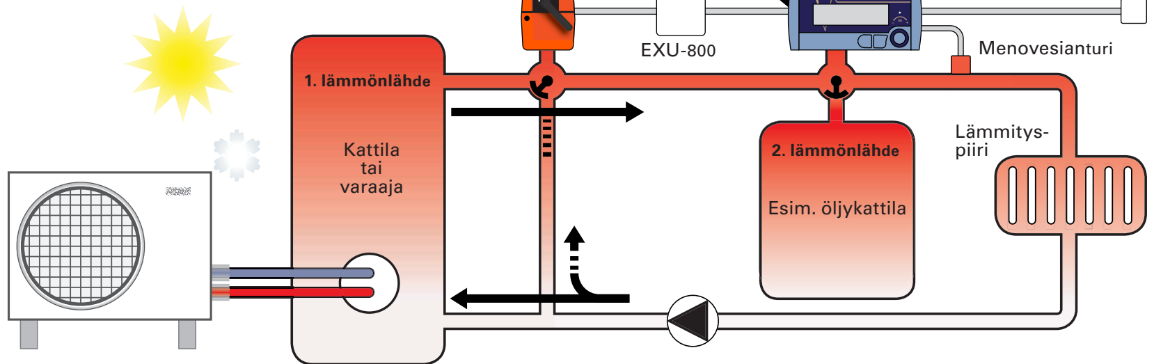
Periaatekuva sarjasäädöstä, lisää periaatekuvia osoitteessa www.ouman.fi
