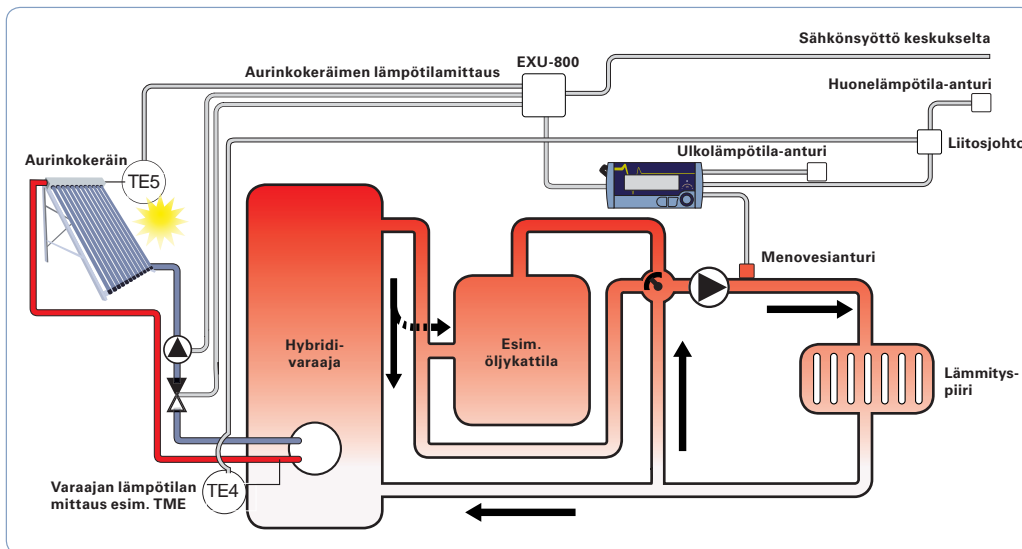
Periaatekuva hybridilämmityksen ohjauksesta, lisää periaatekuvia osoitteessa www.ouman.fi .
