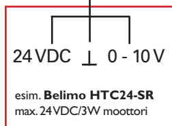
Sarjasäätömoottorin kytkentä EXU-800 laajennusyksikköön
