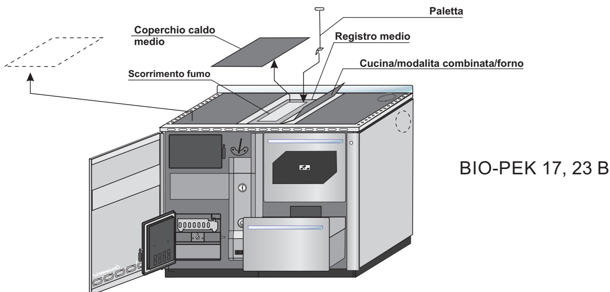
Foto 8. Pulizia – caldaia BIO-PEK B-D (vale anche BIO-PEK B-L)
