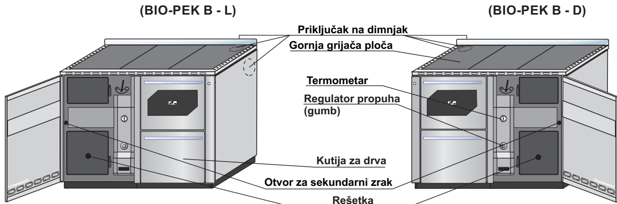
Slika 9. Osnovni dijelovi
