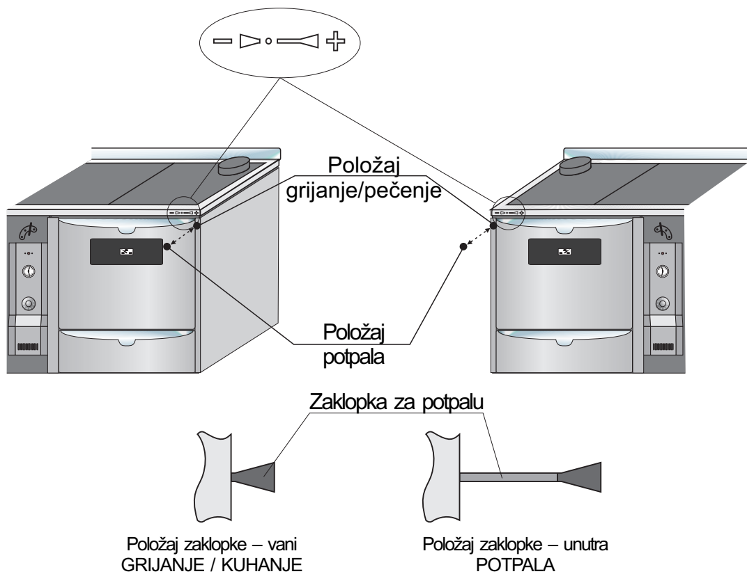
Slika 3. Uporaba zaklopke za potpala kotla BIO-PEK B
