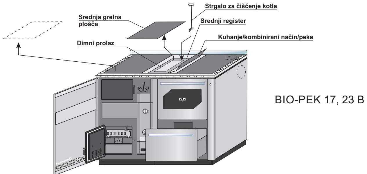
Slika 8. Čiščenje površin – kotel BIO-PEK B–D (velja tudi za kotel BIO-PEK B–L)
