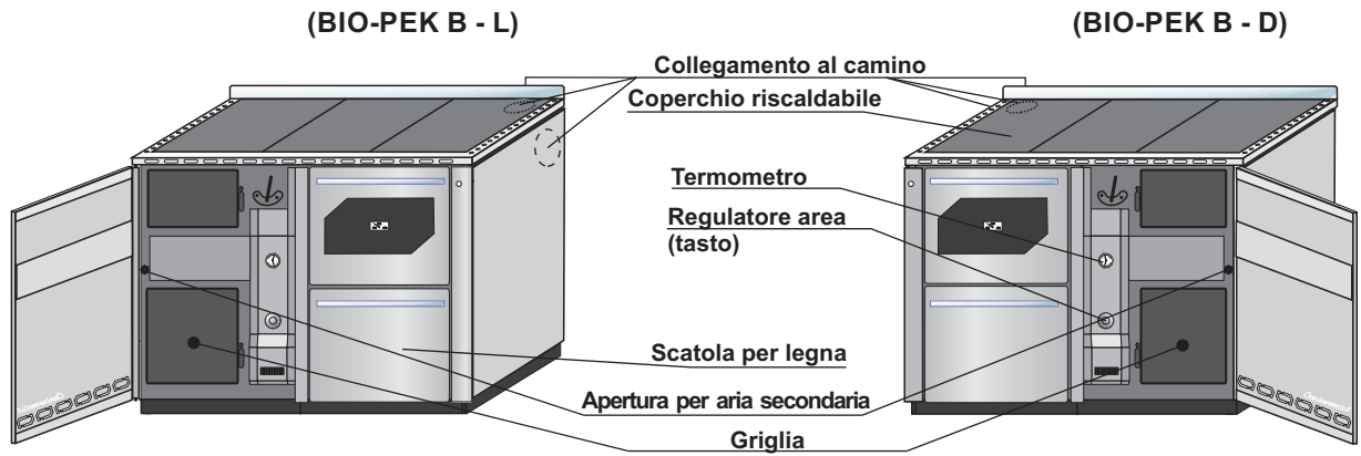
Foto 9. Componente generali
